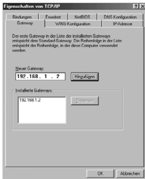
Abbildung 5.2: Eigenschaften von TCP/IP, Gateway
