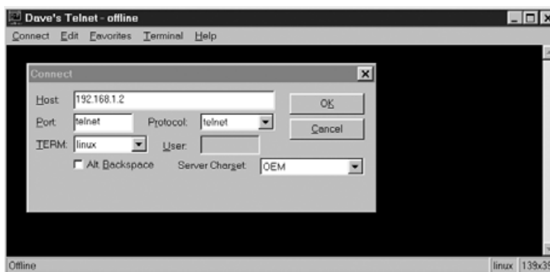
Abbildung 5.11: Anmeldung mit dtelnet
