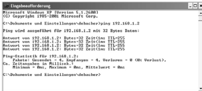
Abbildung 5.4: Ping auf den Server
