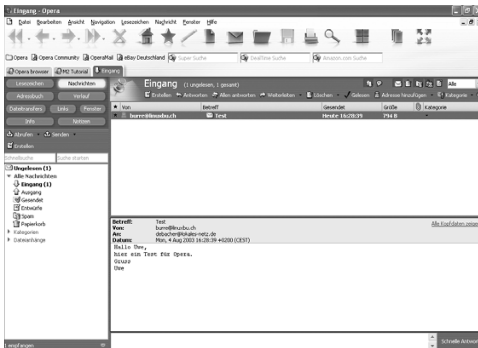
Abbildung 5.56: Opera, einsatzbereit
