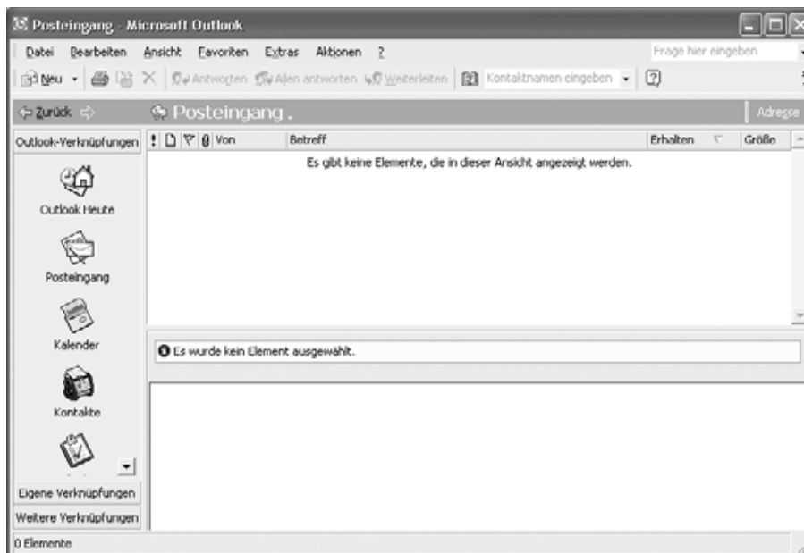
Abbildung 5.23: Outlook 2002, einsatzbereit
