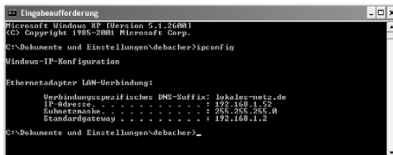
Abbildung 5.7: Ausgabe von ipconfig
