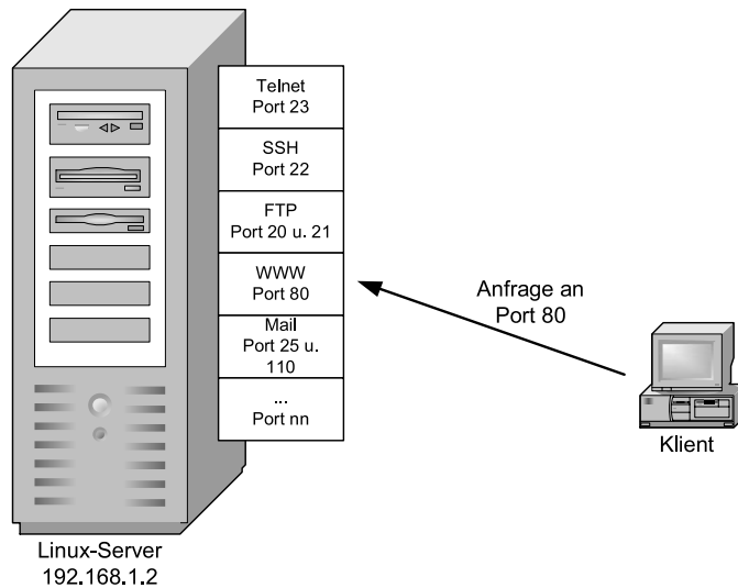
Abbildung 5.9: IP-Adresse und Portnummern
