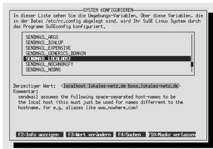
Abbildung 16.5: YaST-System konfigurieren
